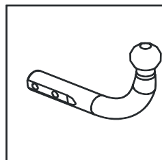
KULA TYP S Kula stała, przykręcana za pomocą dwóch śrub M12
