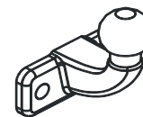
KULA TYP P Płytką z kulą przykręcana za pomocą dwóch śrub M16
